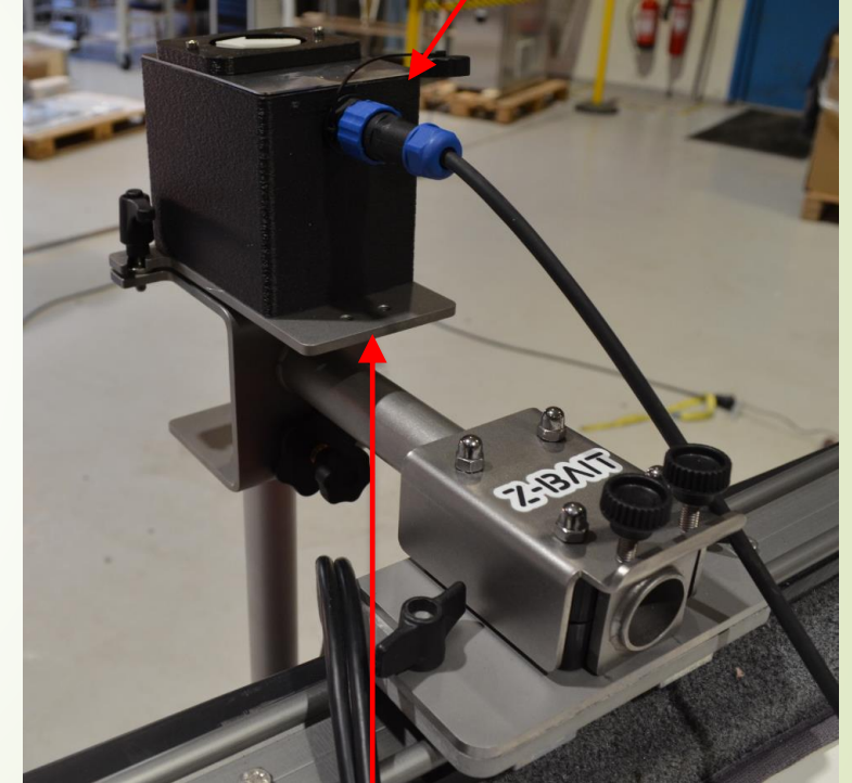
Möjlighet att fästa fast handtag för manuell rotation
